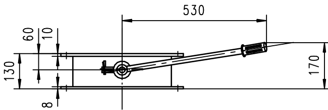
Variante: Auslauf mit Rundflansch
