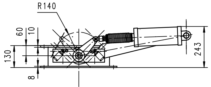
Variante: Auslauf mit Eckflansch
