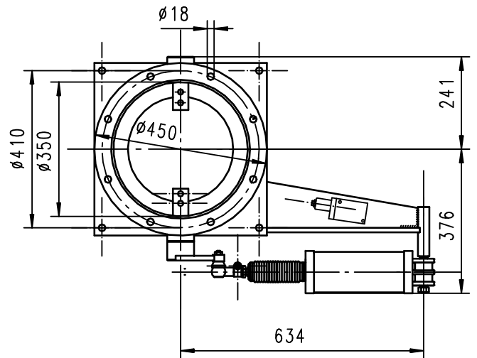
Bohrbild Eckflansch:
