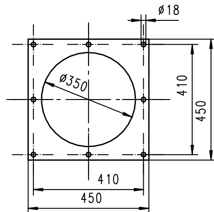
Bohrbild Eckflansch:
