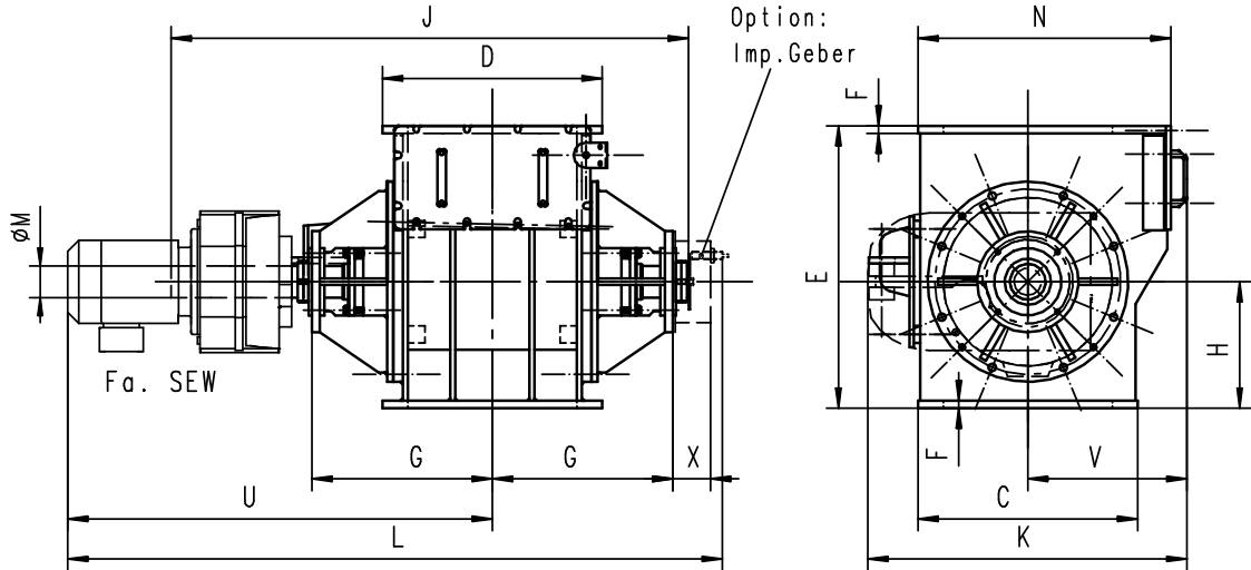
Ansicht A
