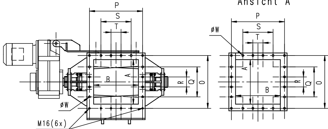
Ansicht A
